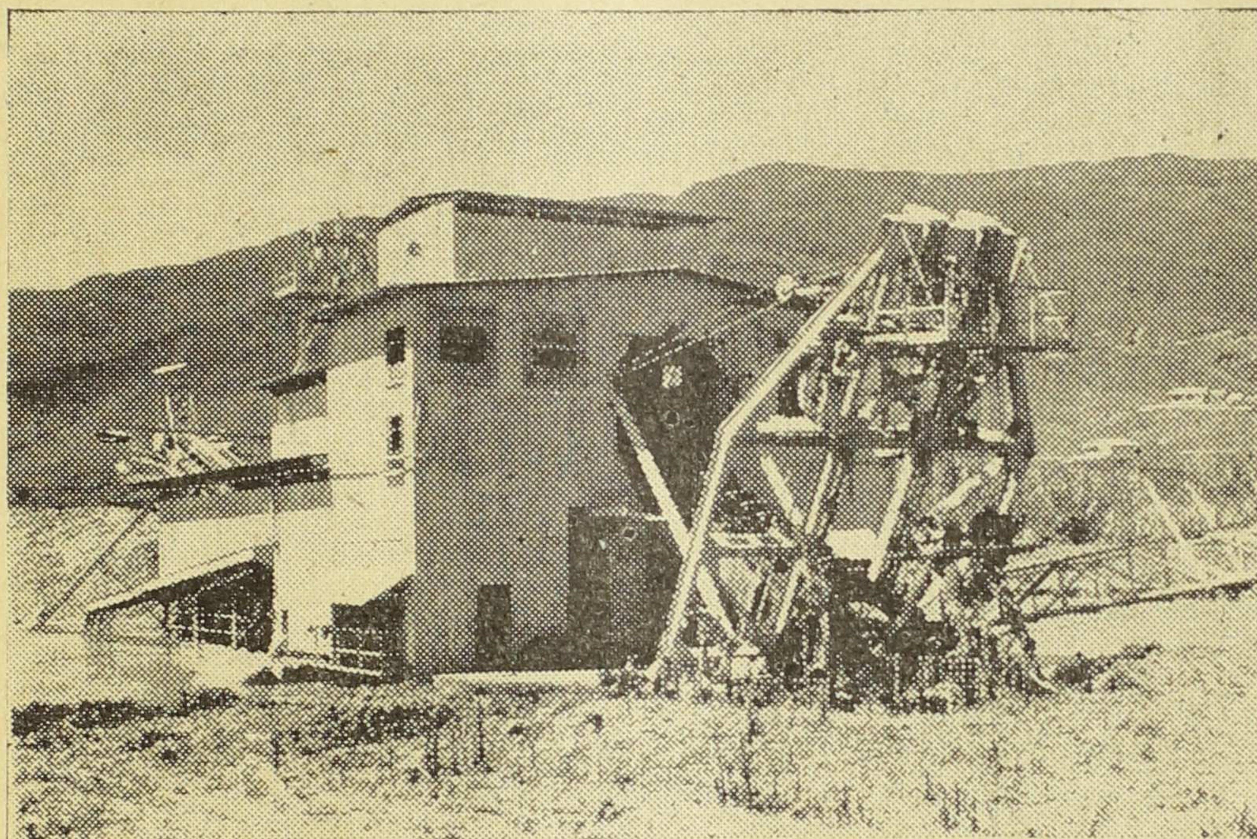
Draga Asnazú número 1, trabajando.
